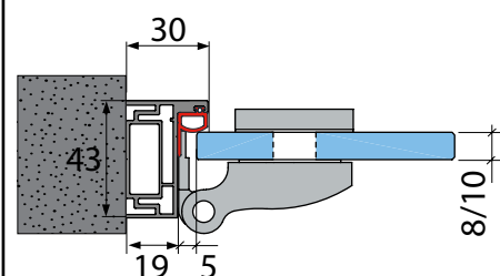
Stipite DV600 anta tuttovetro Installazione in luce
